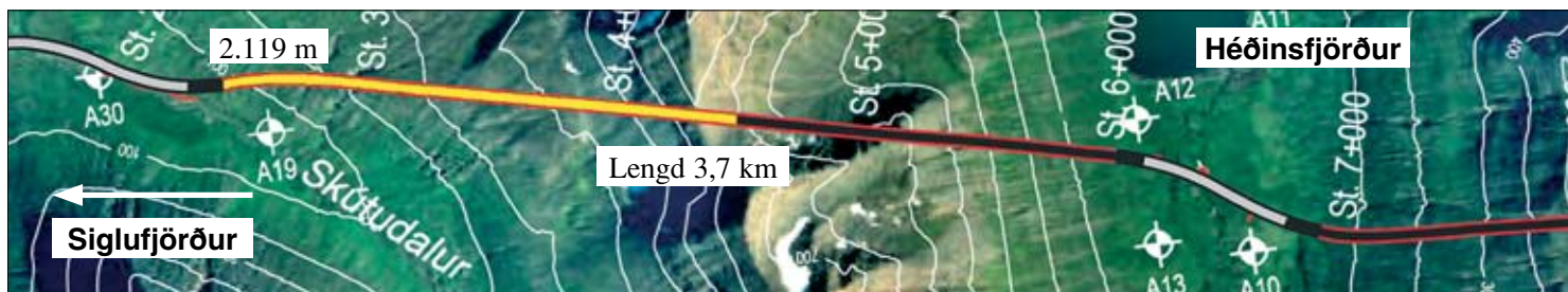
Staða framkvæmda við Héðinsfjarðargöng 6. ágúst 2007. Búið er að sprengja 2.119 m í Siglufirði og 1.646 m í Ólafsfirði.
