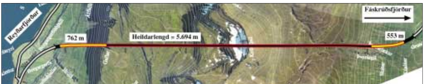
Staða framkvæmda við Fáskrúðsfjarðargöng 21. október 2003. Samtals er búið að sprengja 1.315 m sem gerir 23%.
