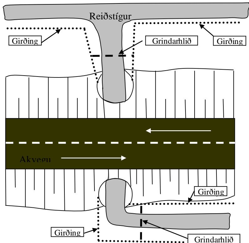
Mynd 6-21 Hugmynd að útfærslu þar sem umferðarlítill reiðleið þverar hjóðveg með mikla umferð og aðstæður þröngar, göng þar sem hugsanlega þarf að teyma í gegn.
