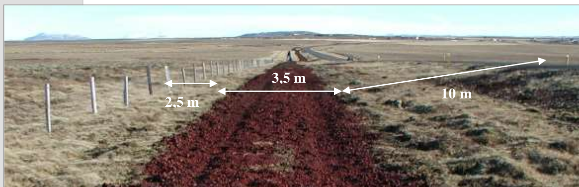
Mynd 6-3 Reiðstígur í Grímsnesi. ADU_{2019} er um 2200 bílar og lega reiðstígsins uppfyllir skilyrði um öryggissvæði vega (hér 10 m) en uppfyllir ekki kröfur um aukið öryggissvæði sem væri hér 15 m. Laus vikur er ekki heppilegt yfirborðsefni reiðstígs.
